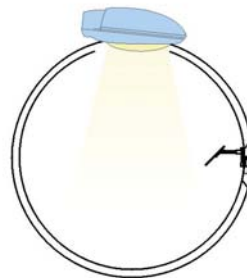
图 3：用积分球测量 LED 路灯的光通量
